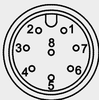
Vue sur l'embase du capteur
